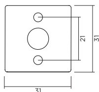
HEXO MINI 1.0
