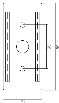
HEXO MINI 2.0
